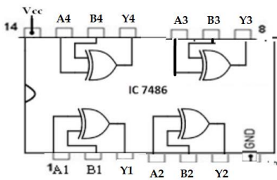
XOR
